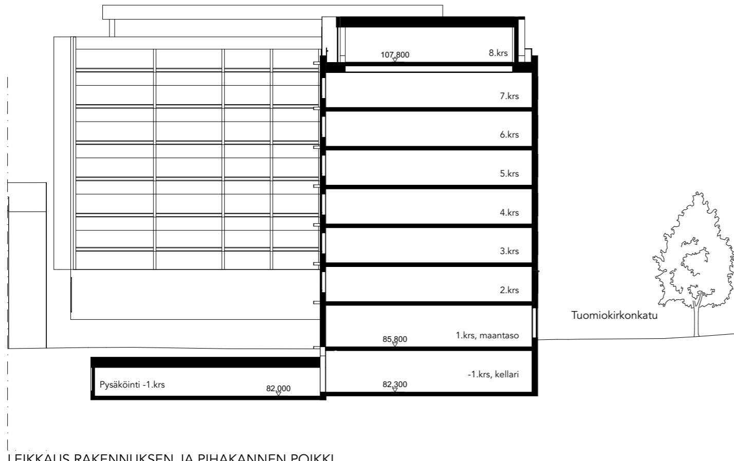
LEIKKAUS RAKENNUKSEN JA PIHAKANNEN POIKKI, KATSELUUNTA POHJOISEEN
